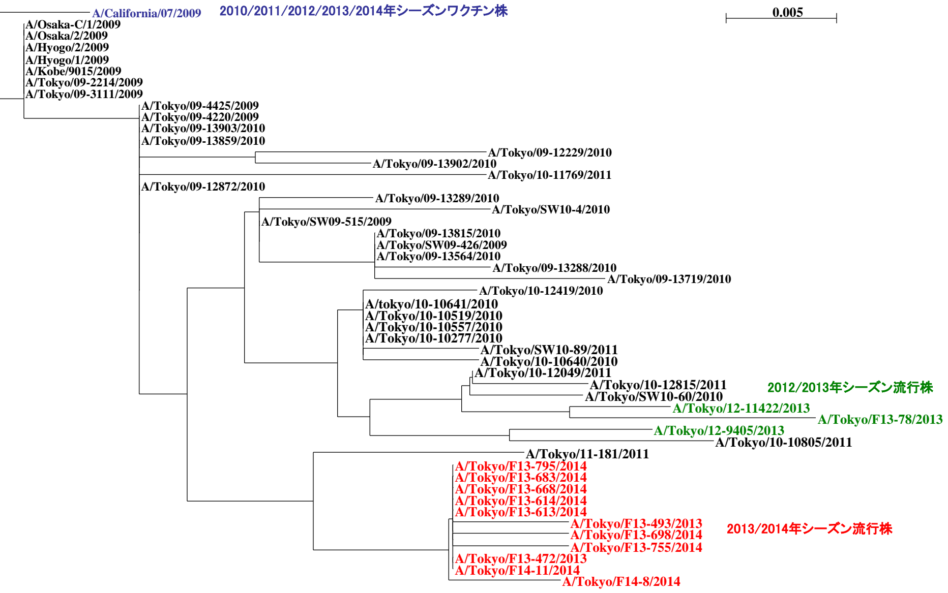
図 東京都におけるAH1pdm09亜型インフルエンザウイルスのHA分子系統樹
