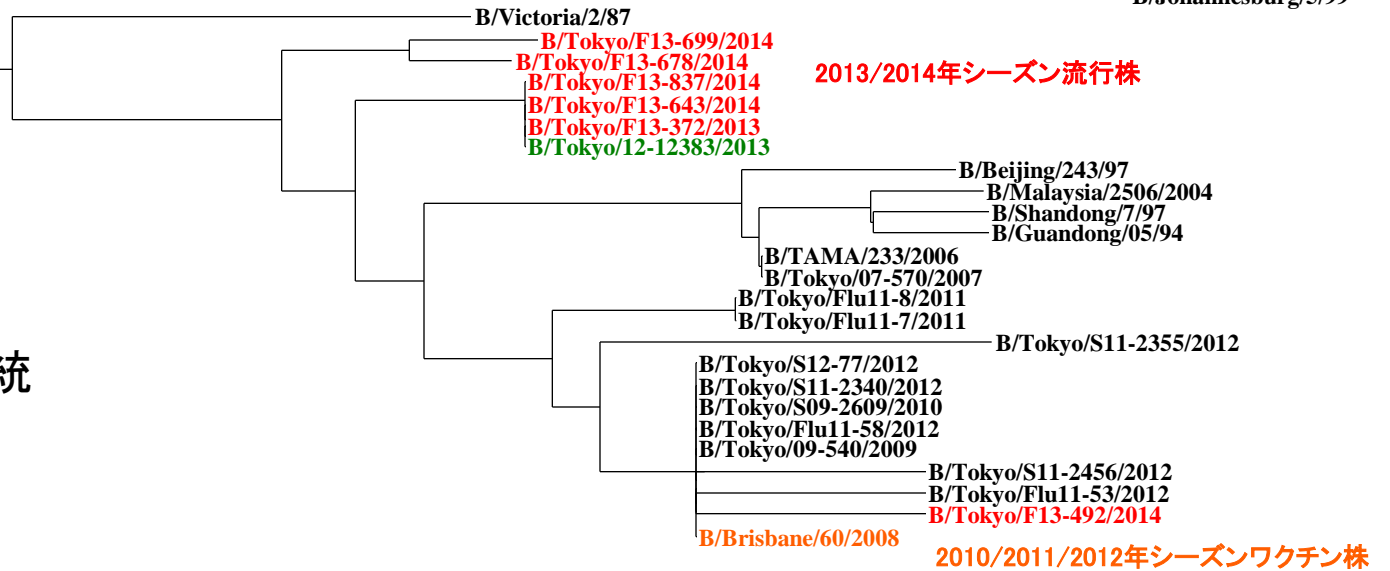
図 東京都におけるB型インフルエンザウイルスのHA分子系統樹
