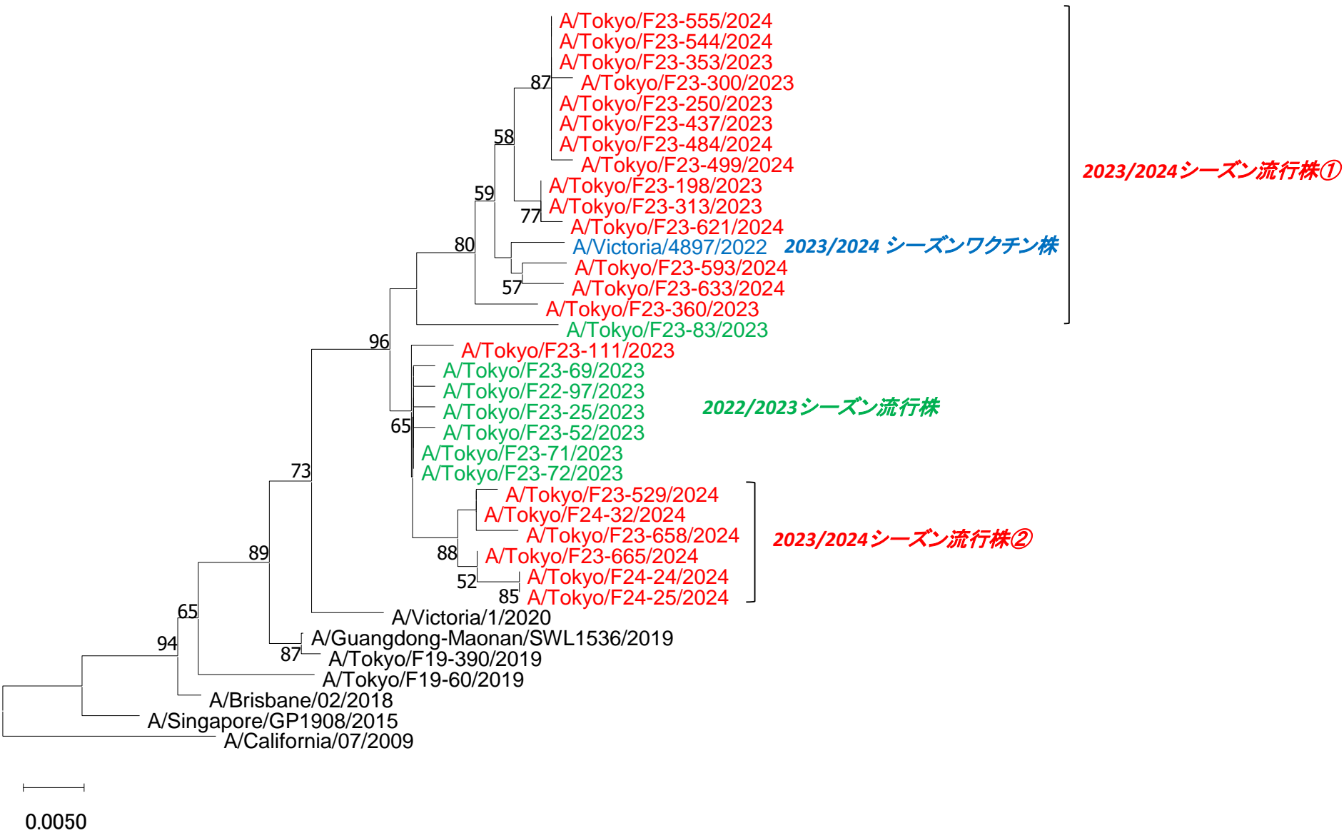
図1. 東京都におけるAH1pdm09インフルエンザウイルスのHA遺伝子系統樹
