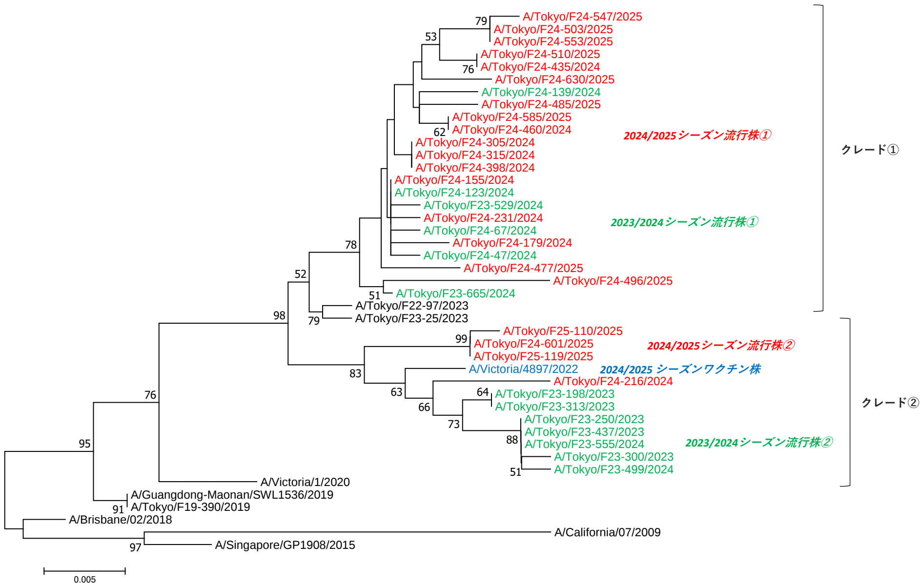
図1. 東京都におけるAH1pdm09インフルエンザウイルスのHA遺伝子系統樹
