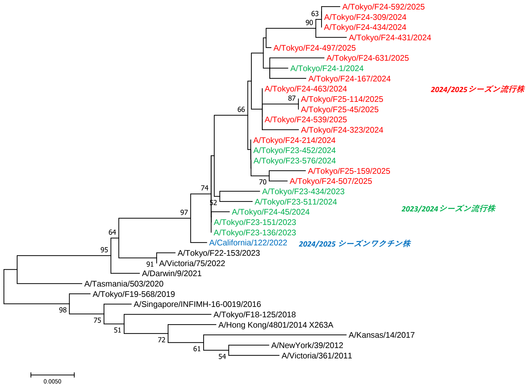
図2. 東京都におけるAH3亜型インフルエンザウイルスのHA遺伝子系統樹
