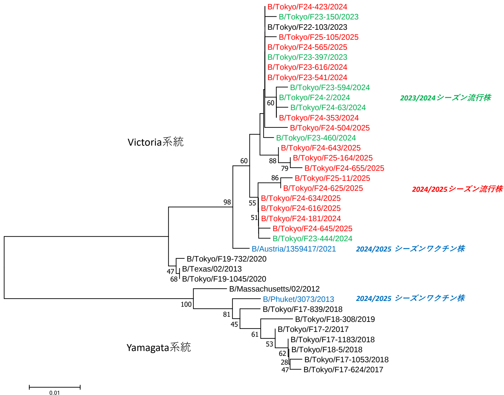
図3. 東京都におけるB型インフルエンザウイルスのHA遺伝子系統樹
