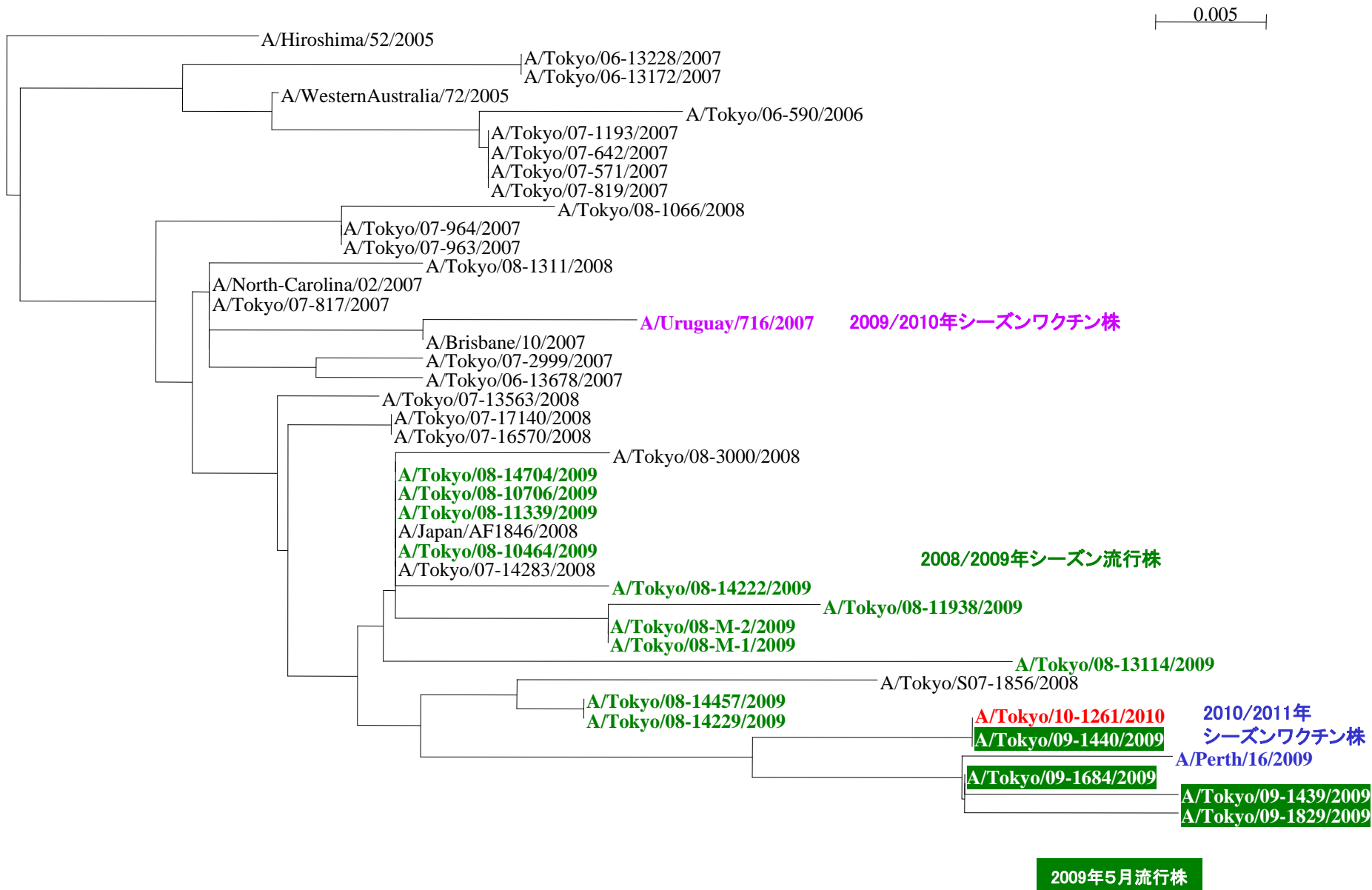
東京都におけるA/H3亜型インフルエンザウイルスのHA遺伝子系統樹
