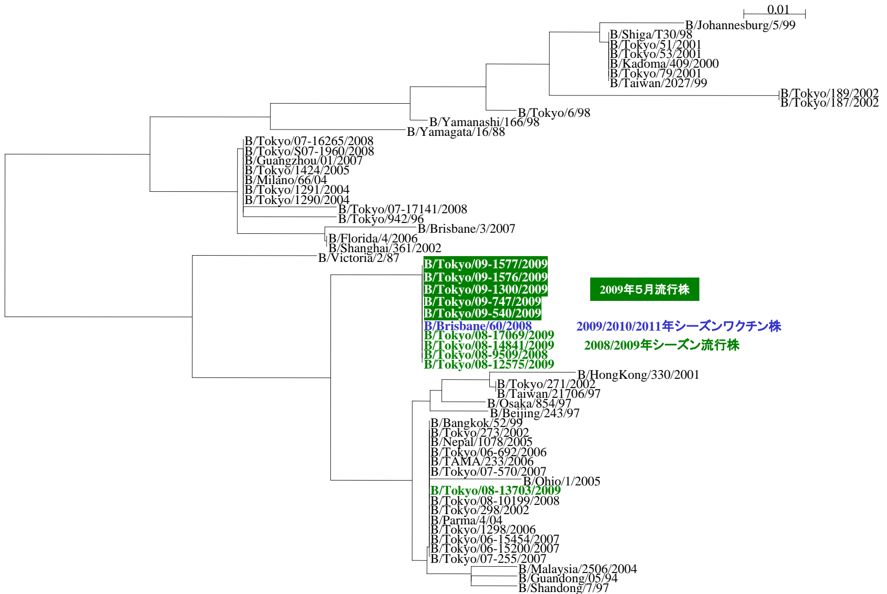
東京都におけるB型インフルエンザウイルスのHA遺伝子系統樹
