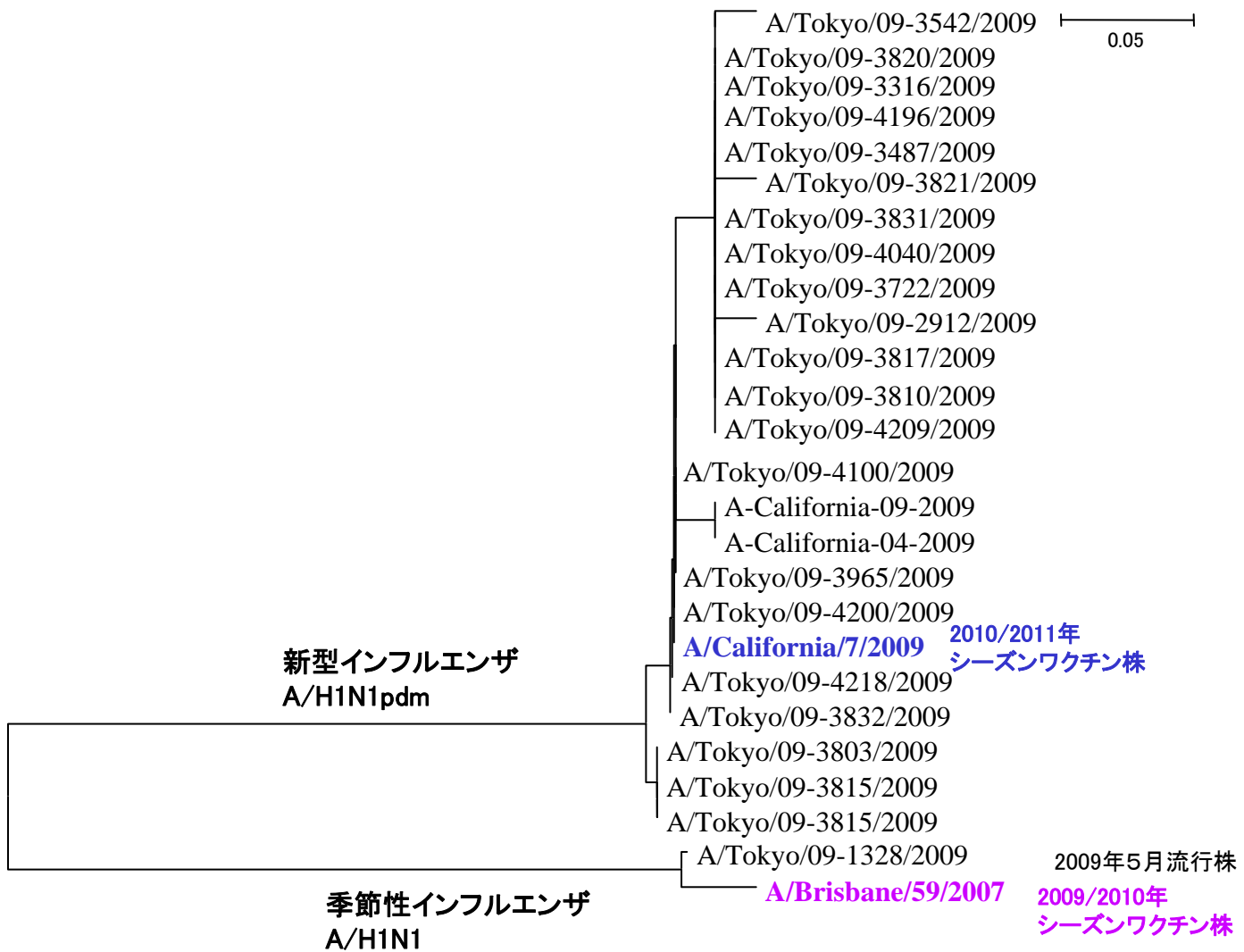
東京都における新型インフルエンザウイルスのHA遺伝子系統樹
